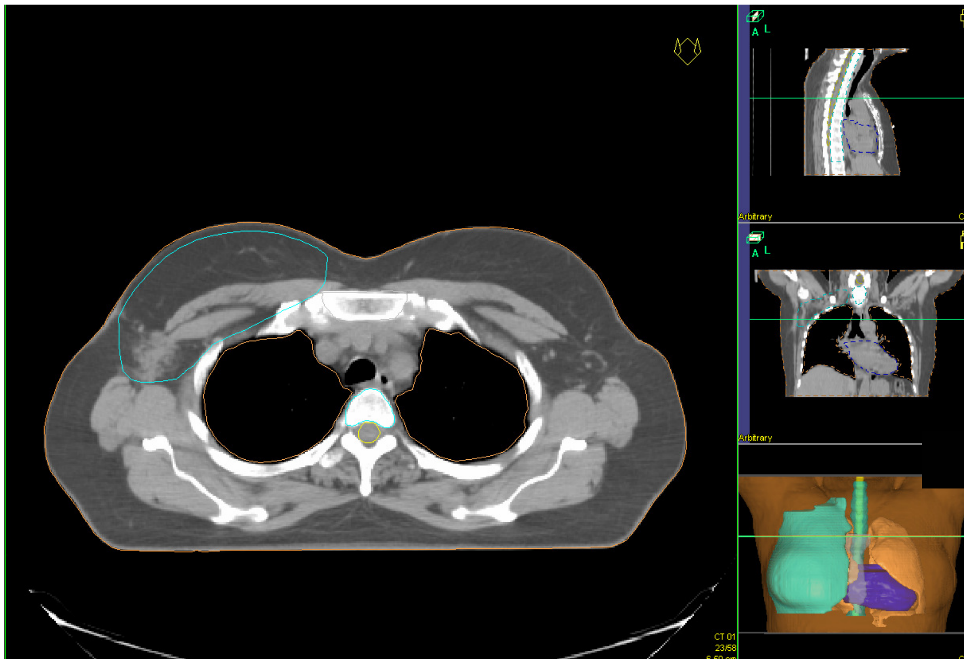
CTV bryst/regionale lymfeknuter inkludert axillenivå I-III
