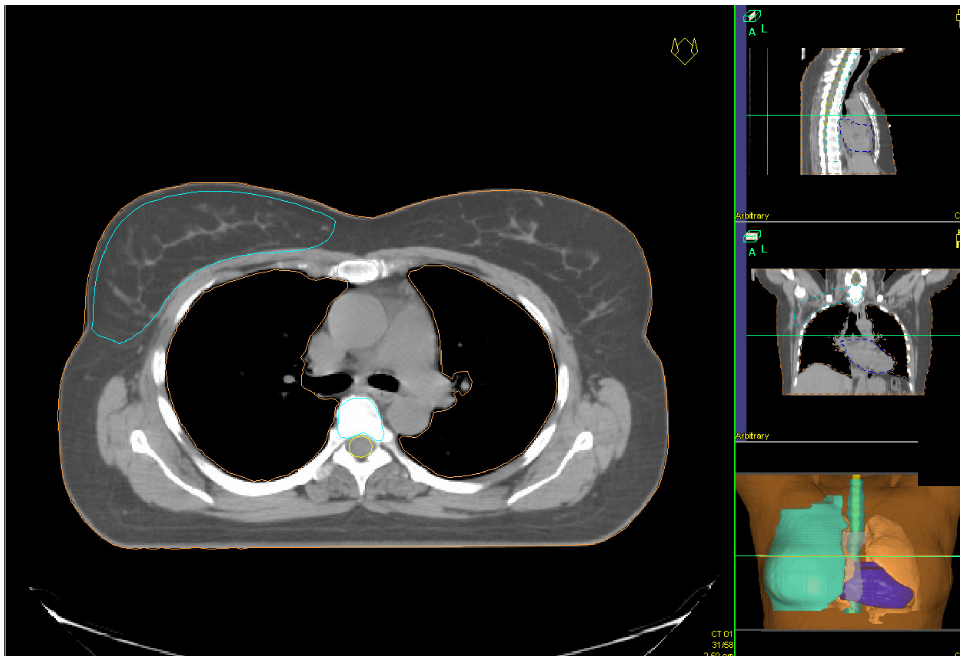
CTV bryst/regionale lymfeknuder inkludert axillenivå I-III
