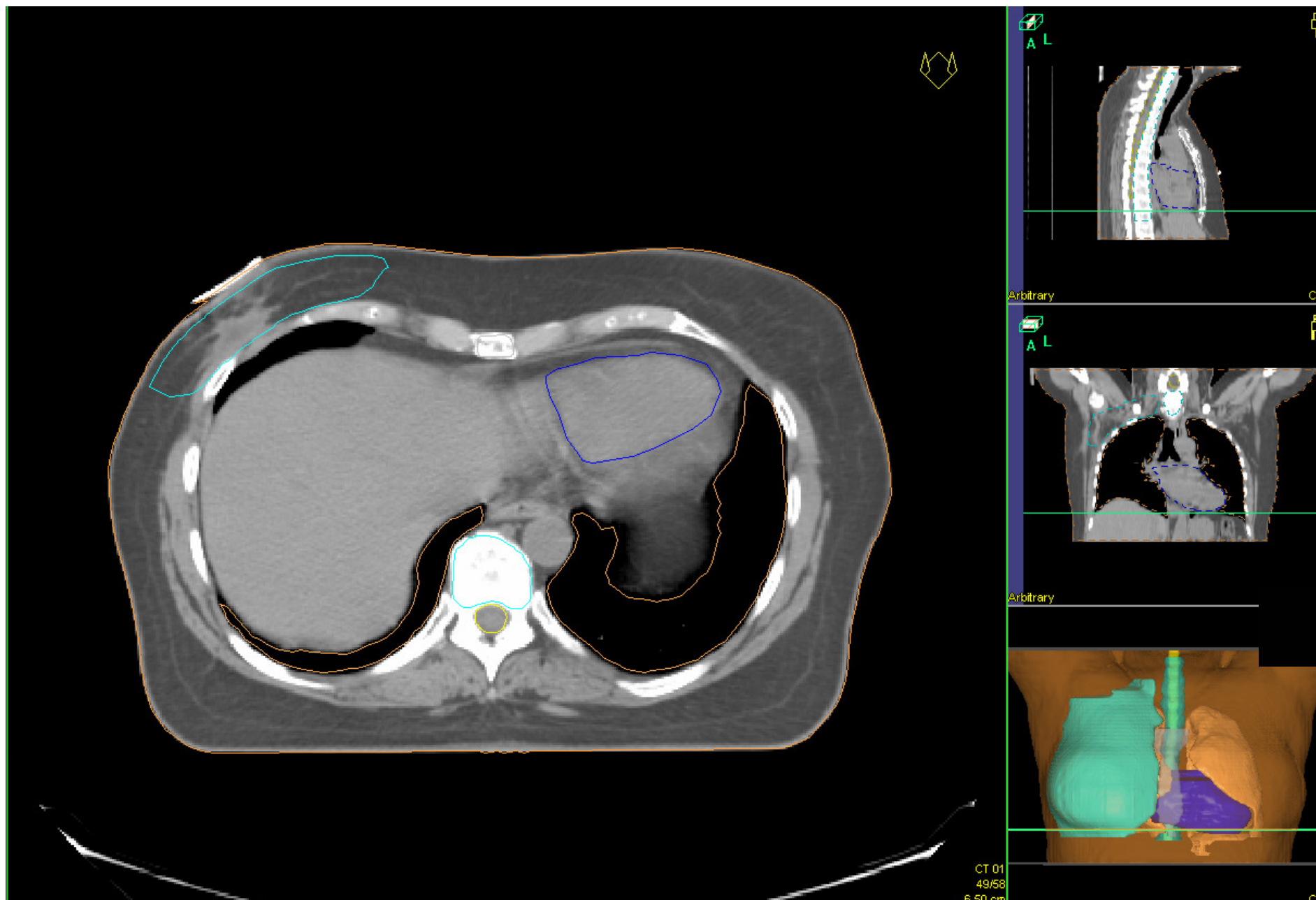
CTV bryst/regionale lymfeknuder inkludert axillenivå I-III
